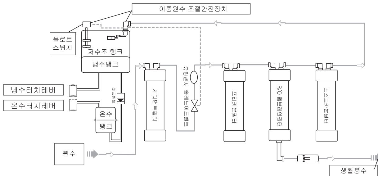
인사이드 케어 수배관도
