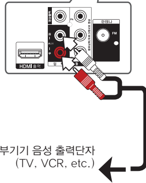
본체의 뒷면
