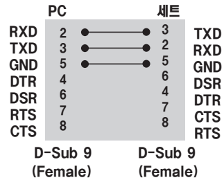
3 와이어 구성(비표준)
