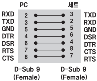
7 와이어 구성(표준 RS-232C 케이블)
