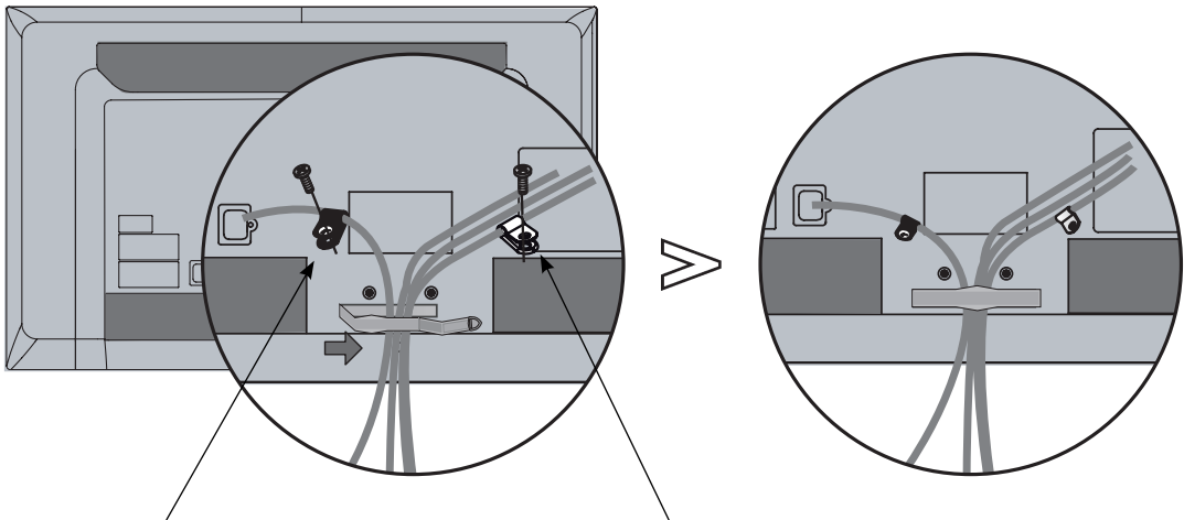
전원코드 홀더(검은색)
