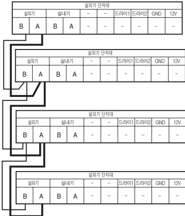
Master 실외기와 Slave 실외기간
