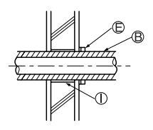
화재 차단벽의 통과 부분과 경계 벽
