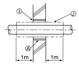
화재 차단벽의 통과 부분과 경계 벽
