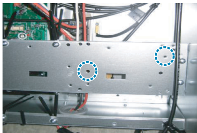
1. C/Box내에 PI-485Gate 장착 Hole를 확인한다.
