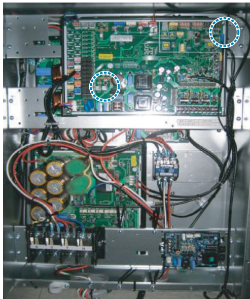
3. Bracket 체결 후 전원선과 통신선을 연결한다.
