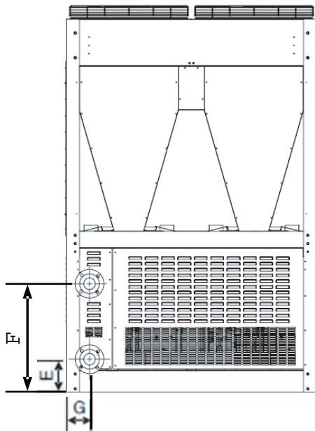
- 후면도 -
