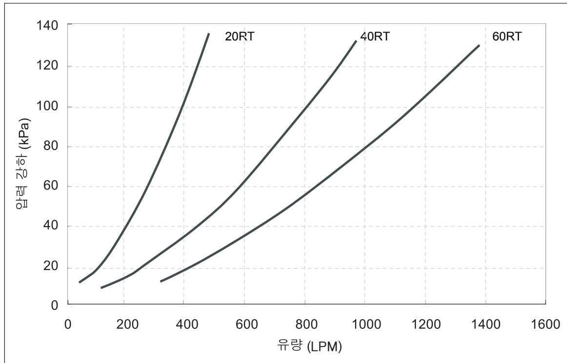
ACHH 시리즈 증발기 수두손실 그래프
