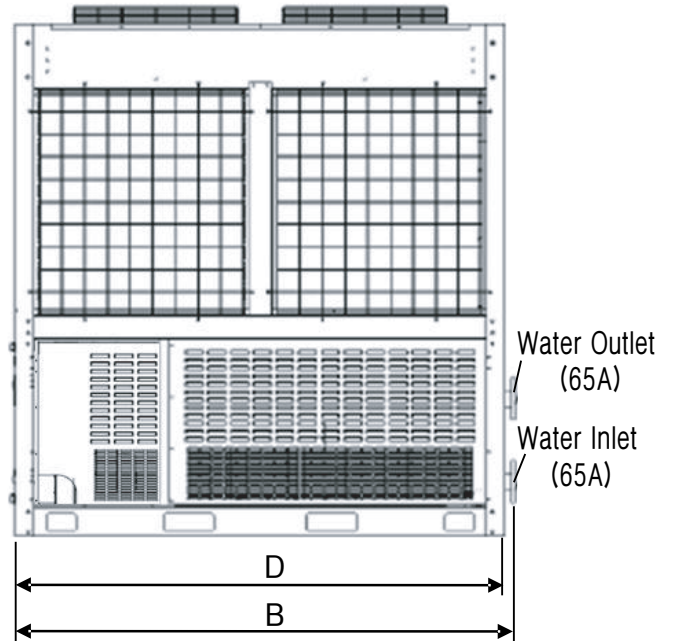
- 측면도 -
