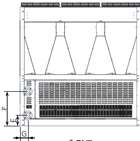
- 후면도 -
