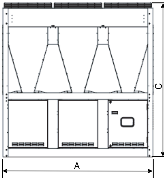
- 정면도 -
