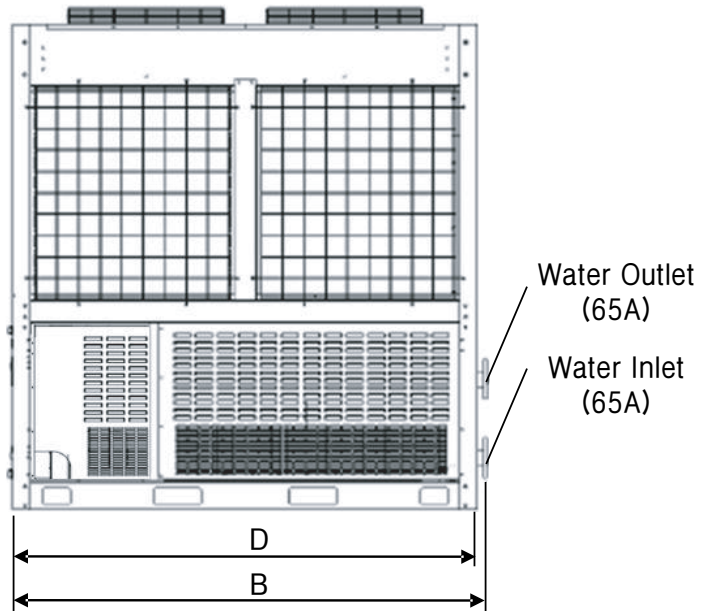
- 측면도 -
